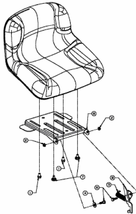
E3-02012A-01
