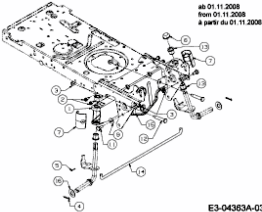
E3-04363A-03
