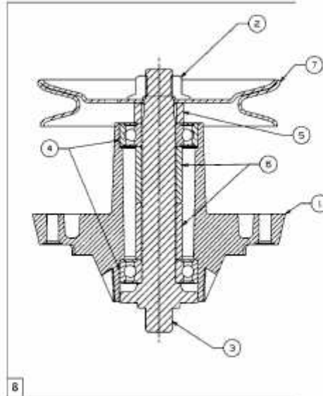
Spindle Assembly / Messerwelle 618-04474
