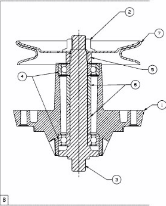
Spindle Assembly / Messerwelle 618-04474
