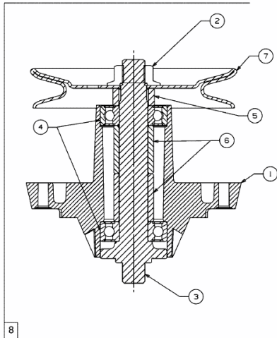
Spindle Assembly / Messerwelle 618-04474
