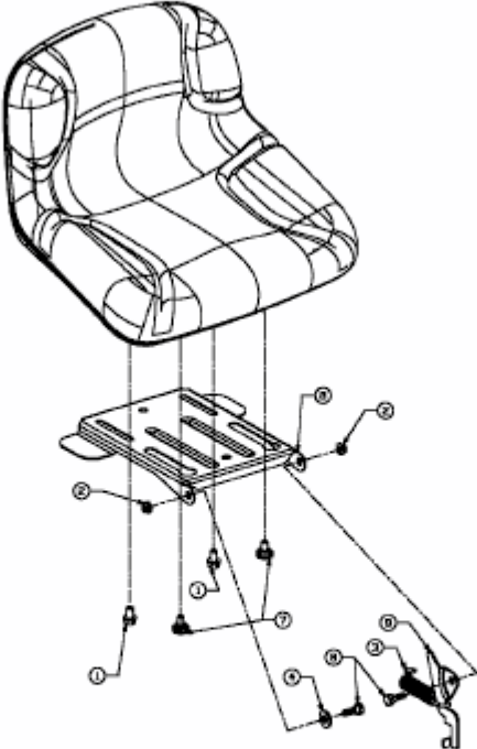
E3-02012A-01
